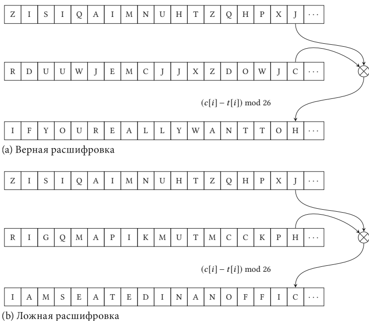
Рисунок 4.9. Одноразовый блокнот, верная и ложная расшифровки
