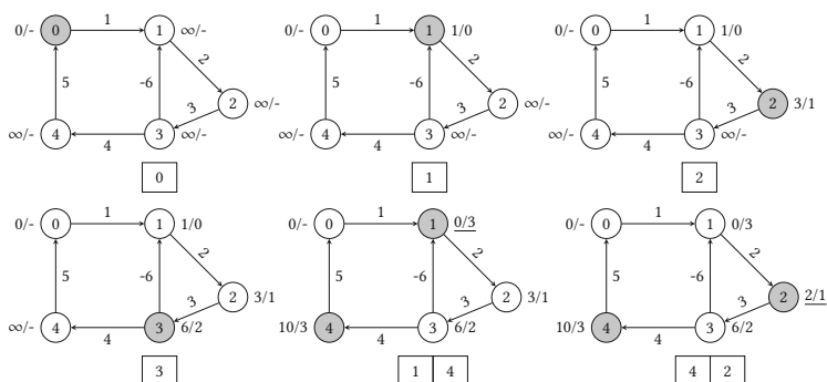
Рисунок 8.10. Ход выполнения алгоритма Беллмана — Форда с отрицательным циклом
