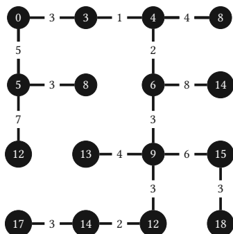
Рисунок 7.8. Связующее дерево дорожной сети
