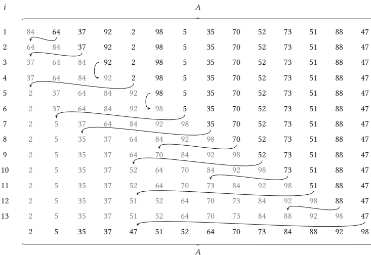
Рисунок 12.3. Пример сортировки методом вставок
