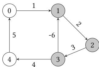
Рисунок 8.9. Граф с отрицательным циклом
