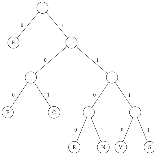
Рисунок 3.6. Код Хаффмана для слова «effervescence»
