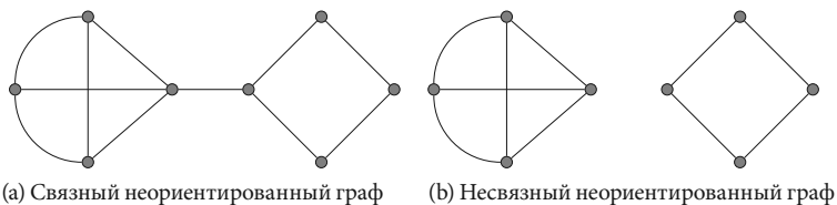
Рисунок 2.6. Неориентированные связные и несвязные графы
