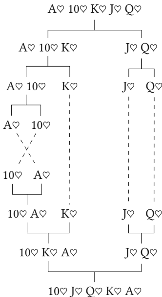
Рисунок 12.13. Сортировка руки с помощью метода слияния
