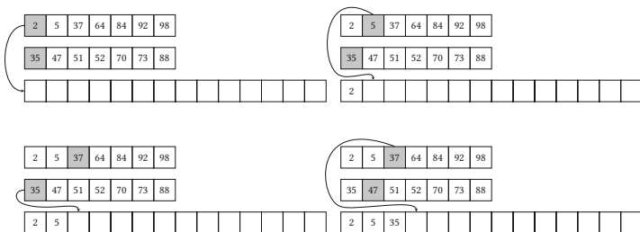
Рисунок 12.11. Слияние двух массивов с помощью указателей
