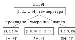
(c) В корневом узле атрибут температуры
