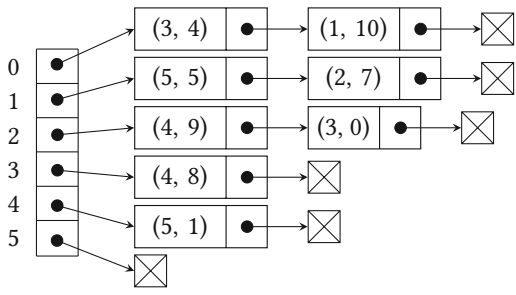
Рисунок 6.7. Представление списка смежности для взвешенного графа с рисунка 6.6
