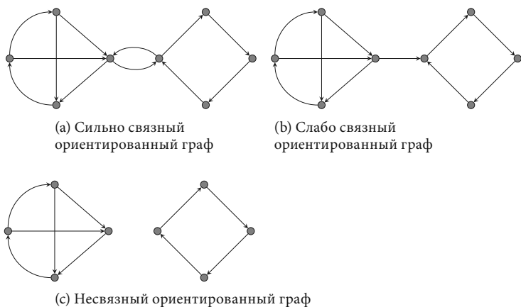
Рисунок 2.7. Связные и несвязные ориентированные графы
