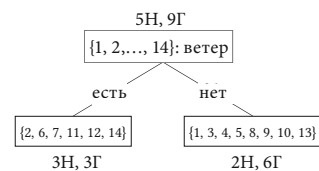
(a) В корневом узле атрибут ветра
