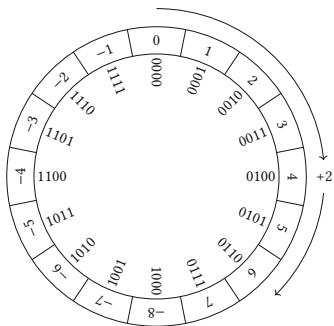
Рисунок 11.19. Вычисление 4 + 2 в дополнительном коде
