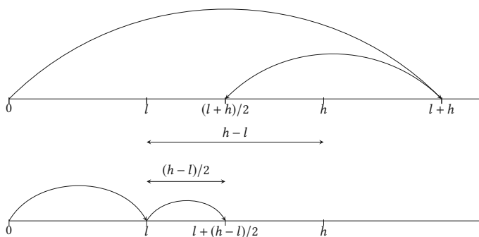
Рисунок 11.22. Избежание переполнения при вычислении срединного числа
