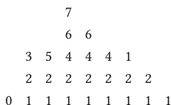
(b) Модификация стека
