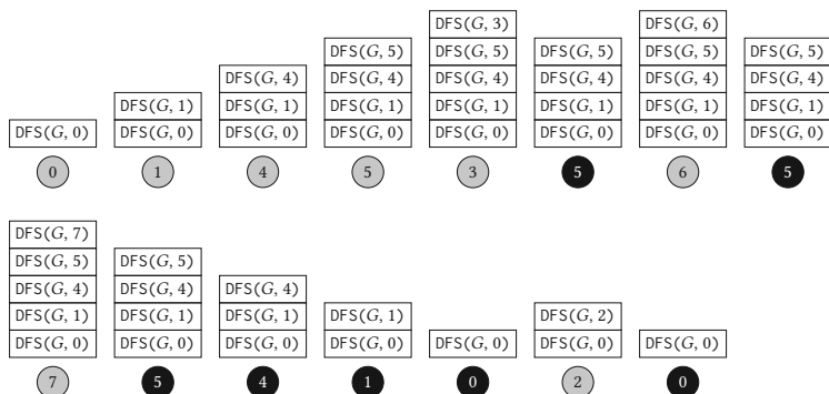
Рисунок 2.24. Поиск в глубину по стеку для рисунка 2.20
