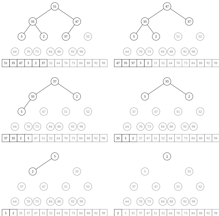
Рисунок 12.8. Вторая фаза сортировки кучей, продолжение
