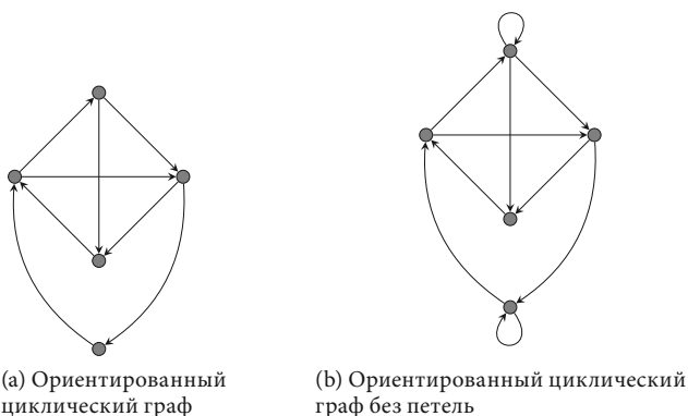
Рисунок 2.8. Циклические ориентированные графы
