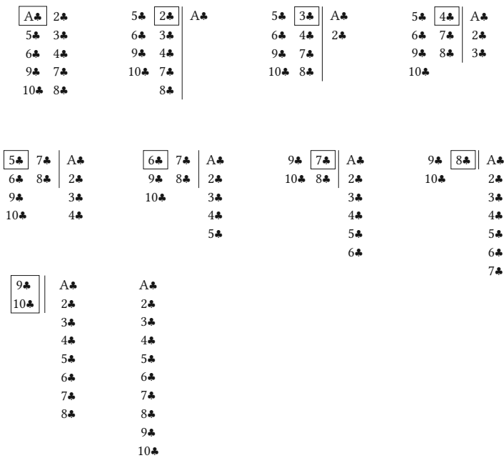
Рисунок 12.9. Слияние двух стопок отсортированных карт
