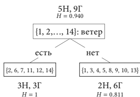
(а) Корневым атрибутом является ветер
