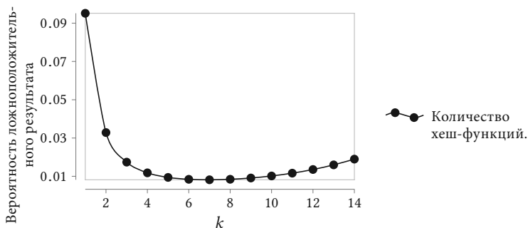
Рисунок 13.18. Вероятность ложноположительного результата в фильтре Блума в виде функции хеш-функций, k , при n/m = 10
