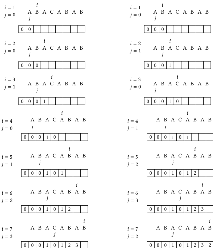
Рисунок 15.7. Ход работы по нахождению границ АВАСАВAB
