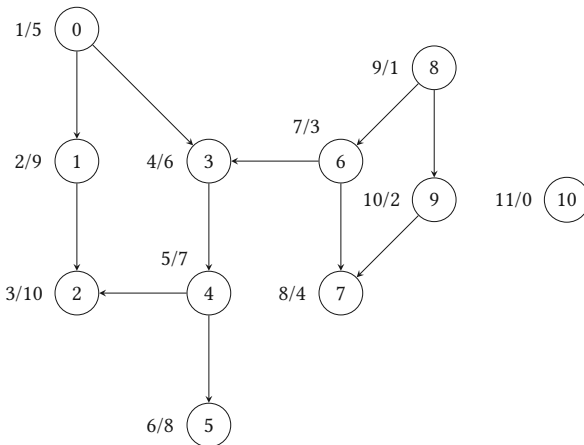
Рисунок 6.4. Обход в глубину графа, отображающего список людей, с топологической сортировкой; отметка i/j рядом с узлом означает, что во время обхода в глубину узел посетили в i порядке, а j указывает место узла в топологической сортировке
