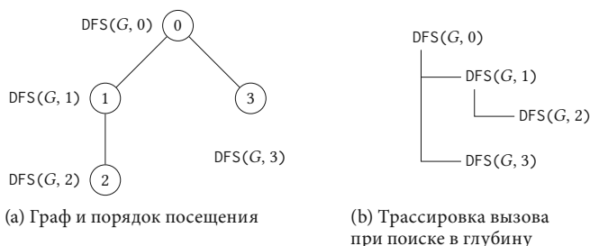
Рисунок 2.21. Углубленный поиск в глубину
