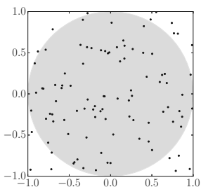
(a) 100 точек, \pi = 3,2 , se = 0,017
