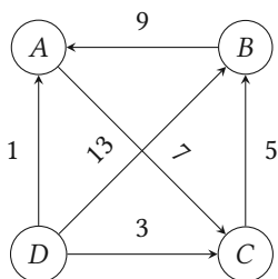
Рисунок 10.1. Граф выборов
