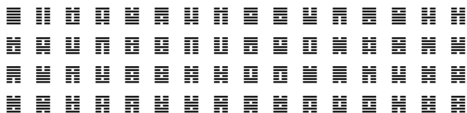
Рисунок 14.1. Гексаграммы «И-Цзин»
