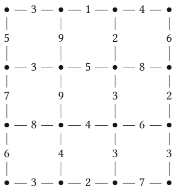
Рисунок 8.4. Дорожная сеть
