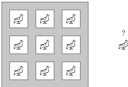
Рисунок 13.2. Принцип Дирихле
