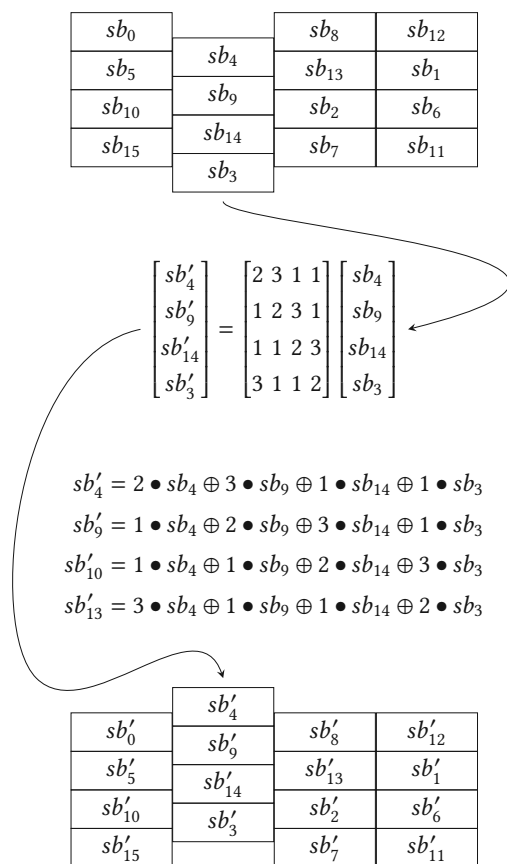
Рисунок 4.14. Операция MixColumns
