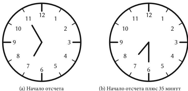
Рисунок 4.7. Добавление минут происходит по модулю 60
