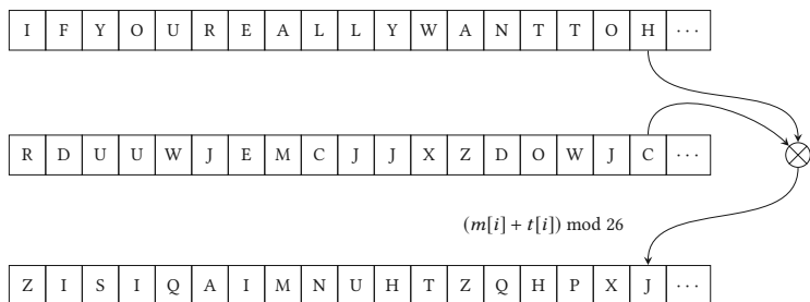
Рисунок 4.8. Одноразовый блокнот
