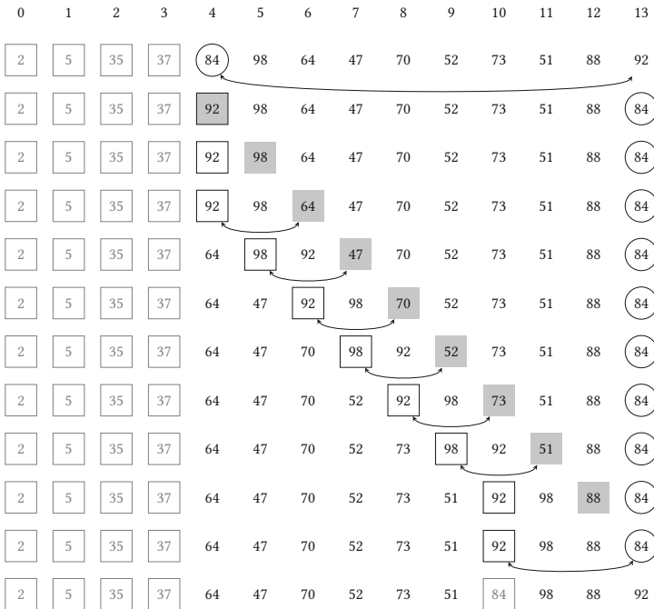
Рисунок 12.17. Пример разделения
