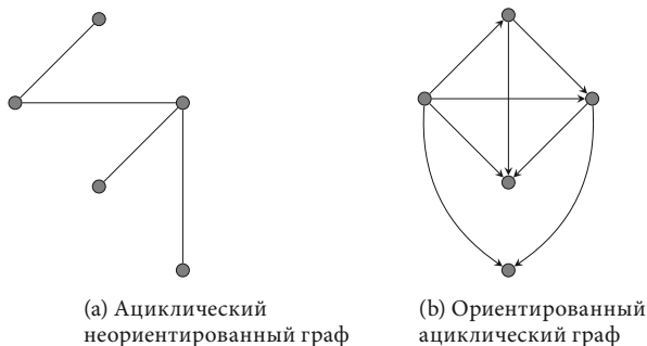
Рисунок 2.9. Ациклические графы
