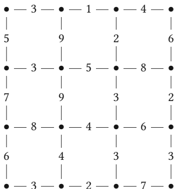
Рисунок 7.5. Дорожная сетка
