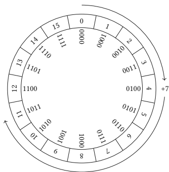
Рисунок 11.16. Вычисление 4 + 7
