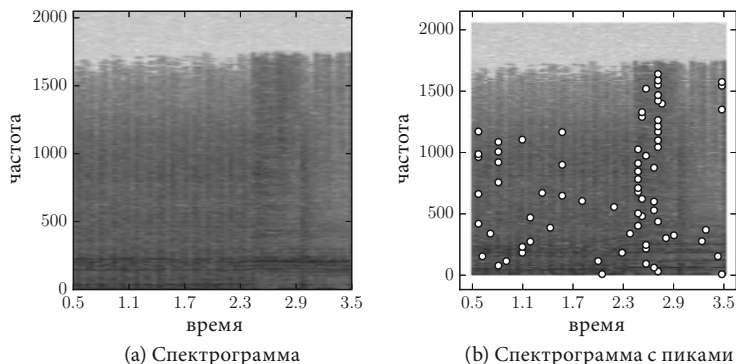
Рисунок 13.14. Спектрограмма и пики мощности частоты
