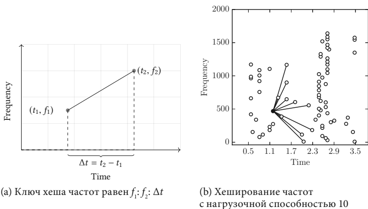
Рисунок 13.15. Пики хеширования частот
