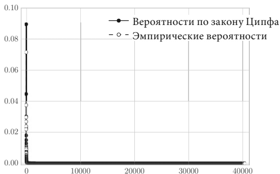
Рисунок 11.6. Эмпирические и теоретические распределения брауновского корпуса
