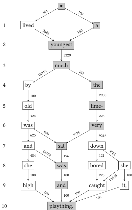
Рисунок 7.3. Оптимизация разрывов строк
