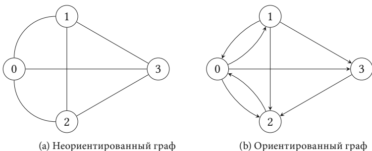
Рисунок 2.5. Ориентированный и неориентированный графы
