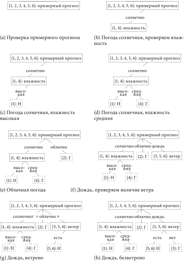
Рисунок 14.6. Этапы построения дерева решений
