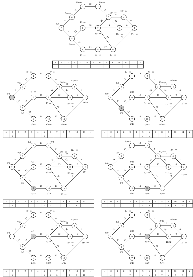
Рисунок 6.13. Нахождение критического пути. Отметка i/j рядом с узлом означает, что узел имеет топологический порядок i и расстояние j . Матрица под каждым изображением показывает pred с пустыми элементами вместо -1 , чтобы уменьшить лишние скопления
