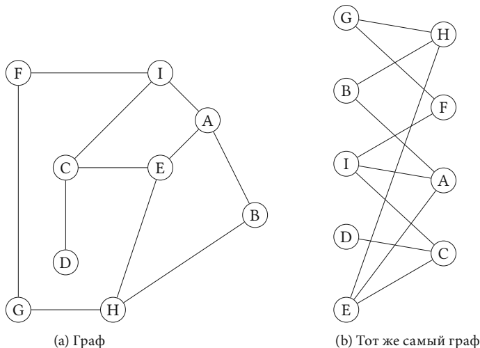
Рисунок 2.10. Двудольный граф
