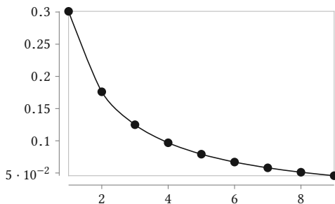
Рисунок 11.8. Закон Бенфорда
