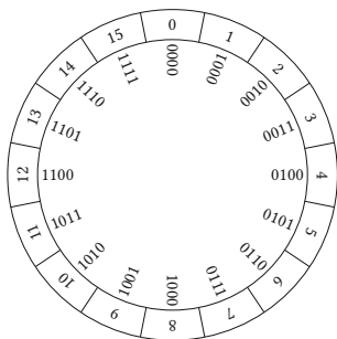
Рисунок 11.15. Числовое колесо
