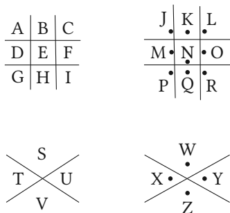
Рисунок 4.6. Масонский шифр
