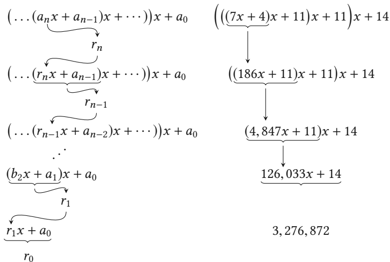
Рисунок 13.5. Схема Горнера
