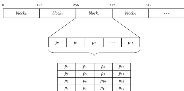
Рисунок 4.10. AES-операция CreateState
