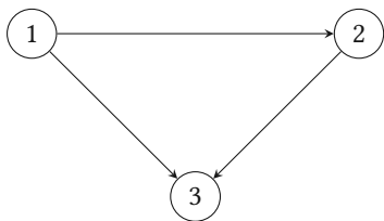
Рисунок 9.3. Проседание пейдж-ранка
