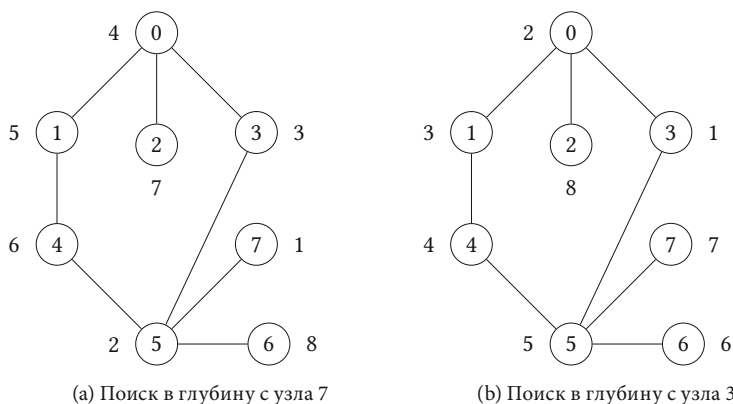
Рисунок 2.23. Исследование в глубину с различных узлов
